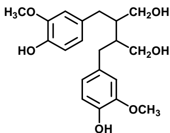
Secoisolariciresinol
