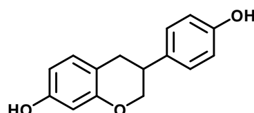
Equol
