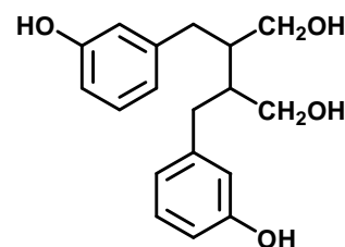
Enterodiols
