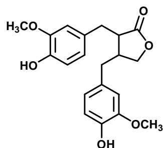
Matairesinol
