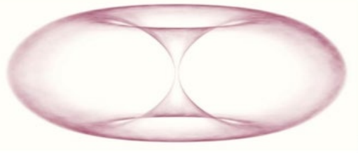
FIG.2.1. The Universal torus
