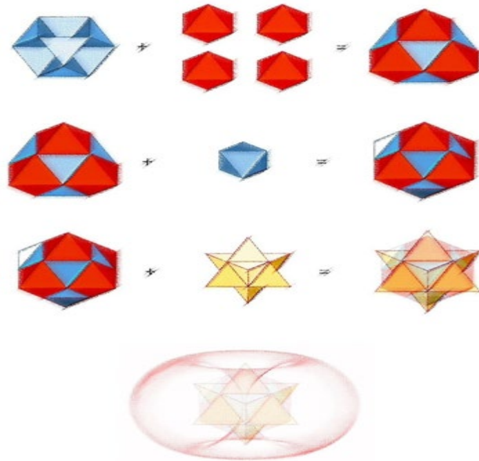
FIG. 3.4 - The Electron (-1)
