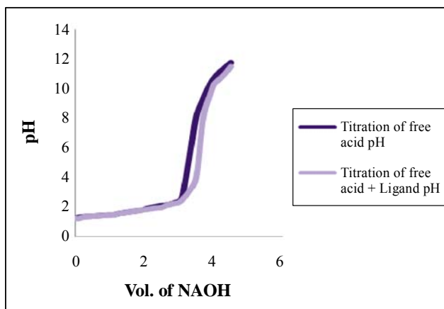
Fig. 3: System: HNMP2FI L3
