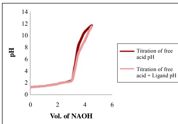
Fig. 2: System: HNMP4CI L2
