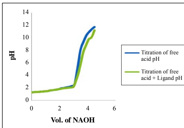
Fig. 1: System: HNMP3NI L1
